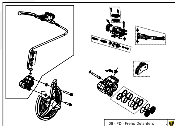
08-FD-Freno Delantera
