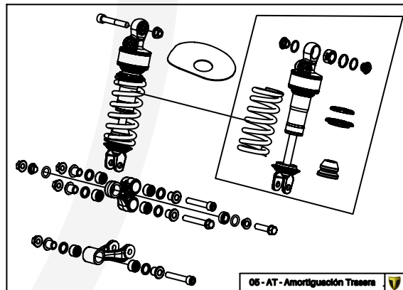
06-AT-Amortiguación Trasera
